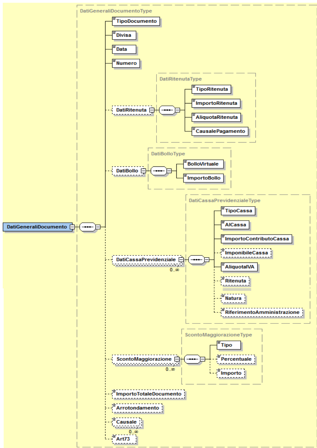
Figura 19: Elemento DatiGeneralDocumento
